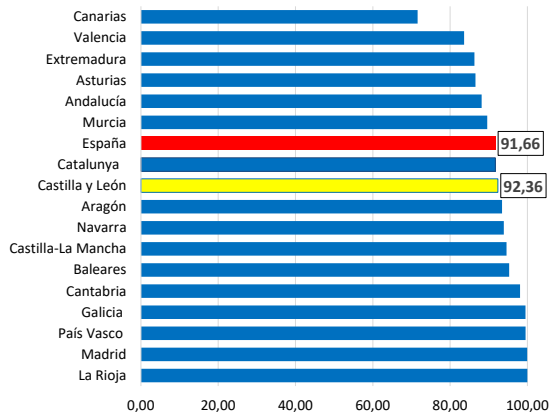
Solicitudes resueltas (%)
