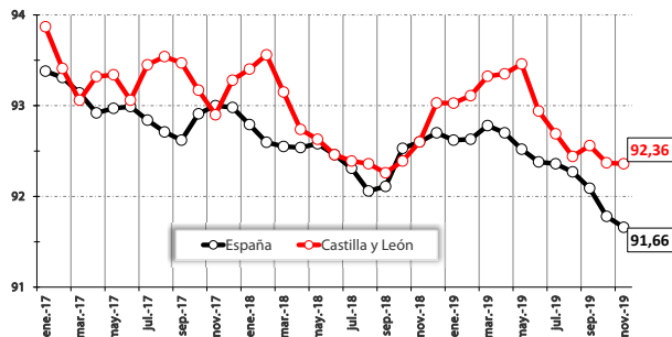
Solicitudes resueltas (%)
