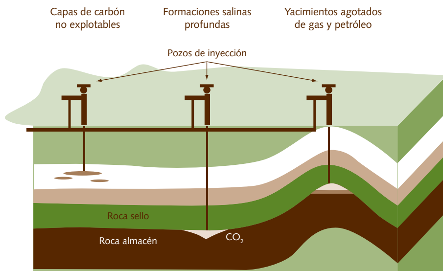
Figura 2.35 Tipos de almacenes geológicos
