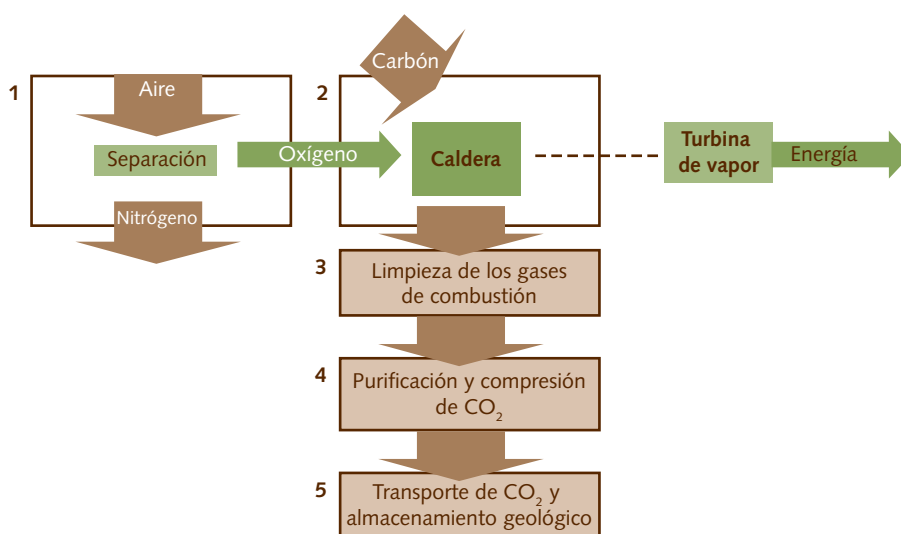
Figura 2.34 Diagrama de flujo de los procesos de oxicomcombustión y captura de CO 2
