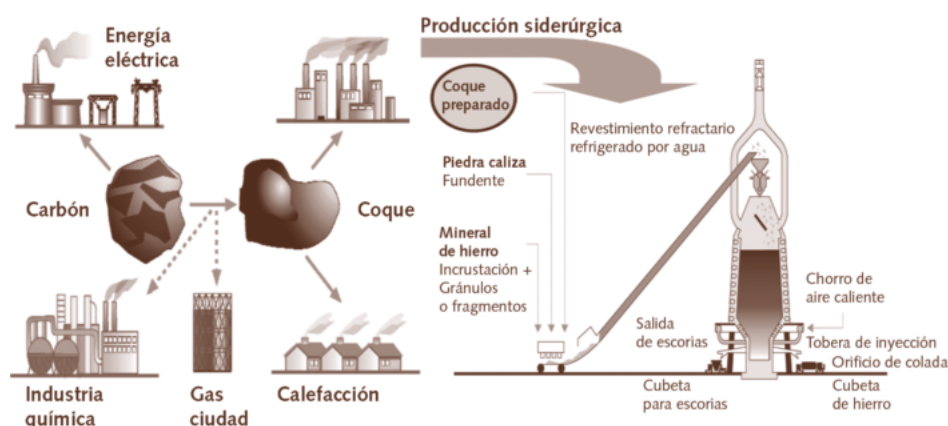
Figura 2.1 Esquema básico de usos de las tecnologías del carbón
